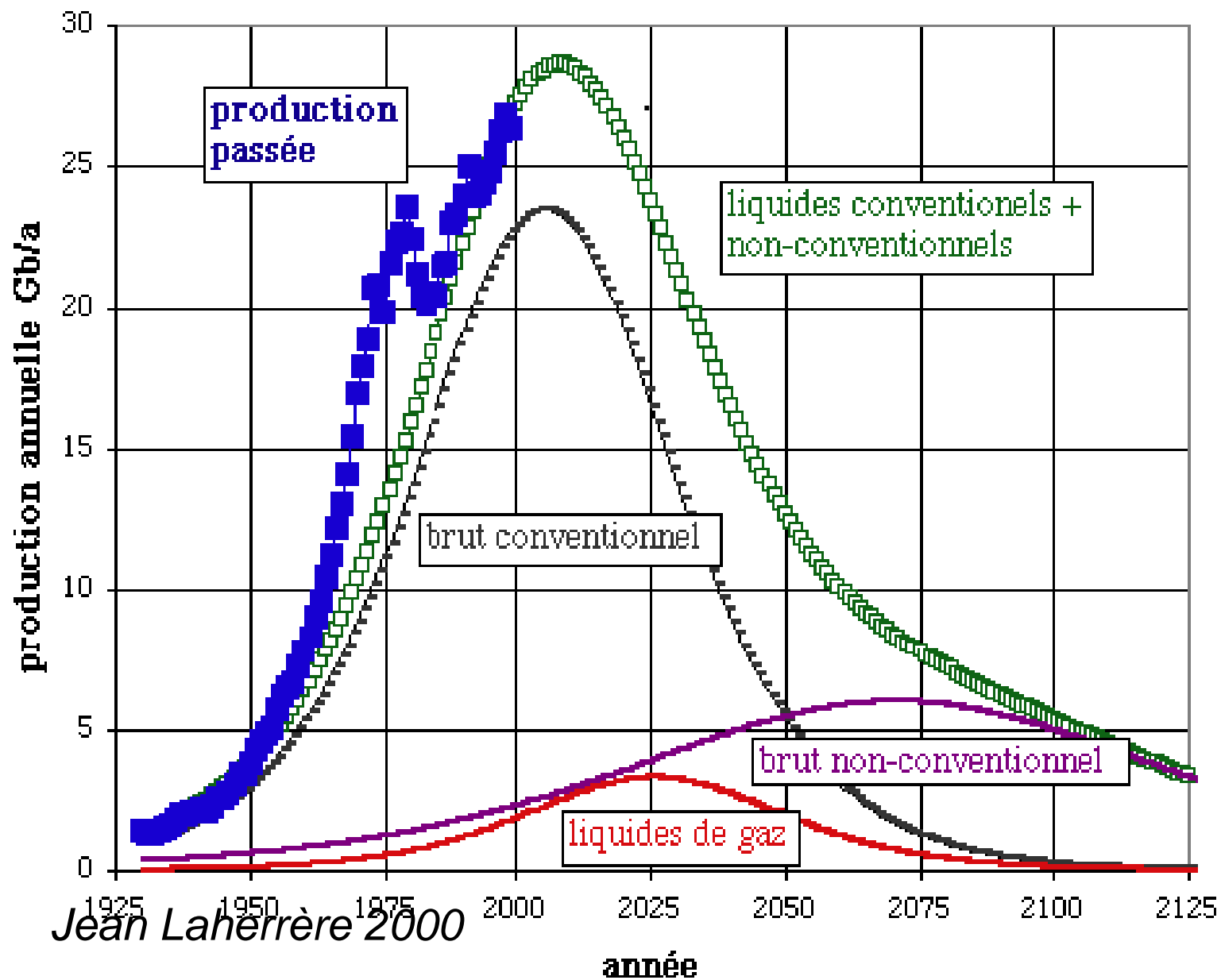
Production mondiale des liquides: ultime 2000 Gb conventionnel + 750 Gb non-conventionnel
